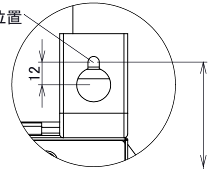
詳細図 A 上部本体固定穴詳細図 (スケール 1 : 2)
