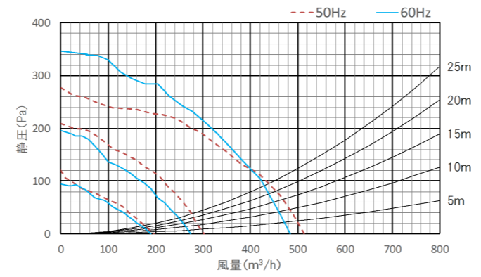
■静圧・風量・性能表
